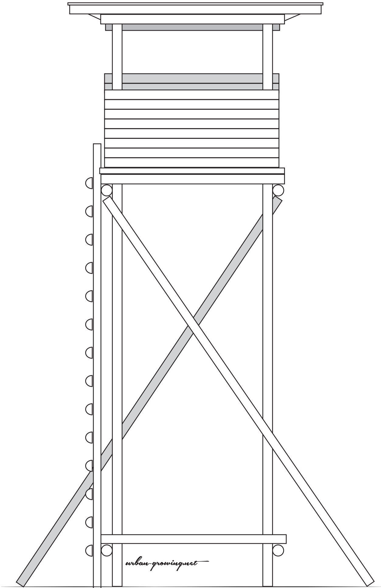
EINFACHER WACHTURM
