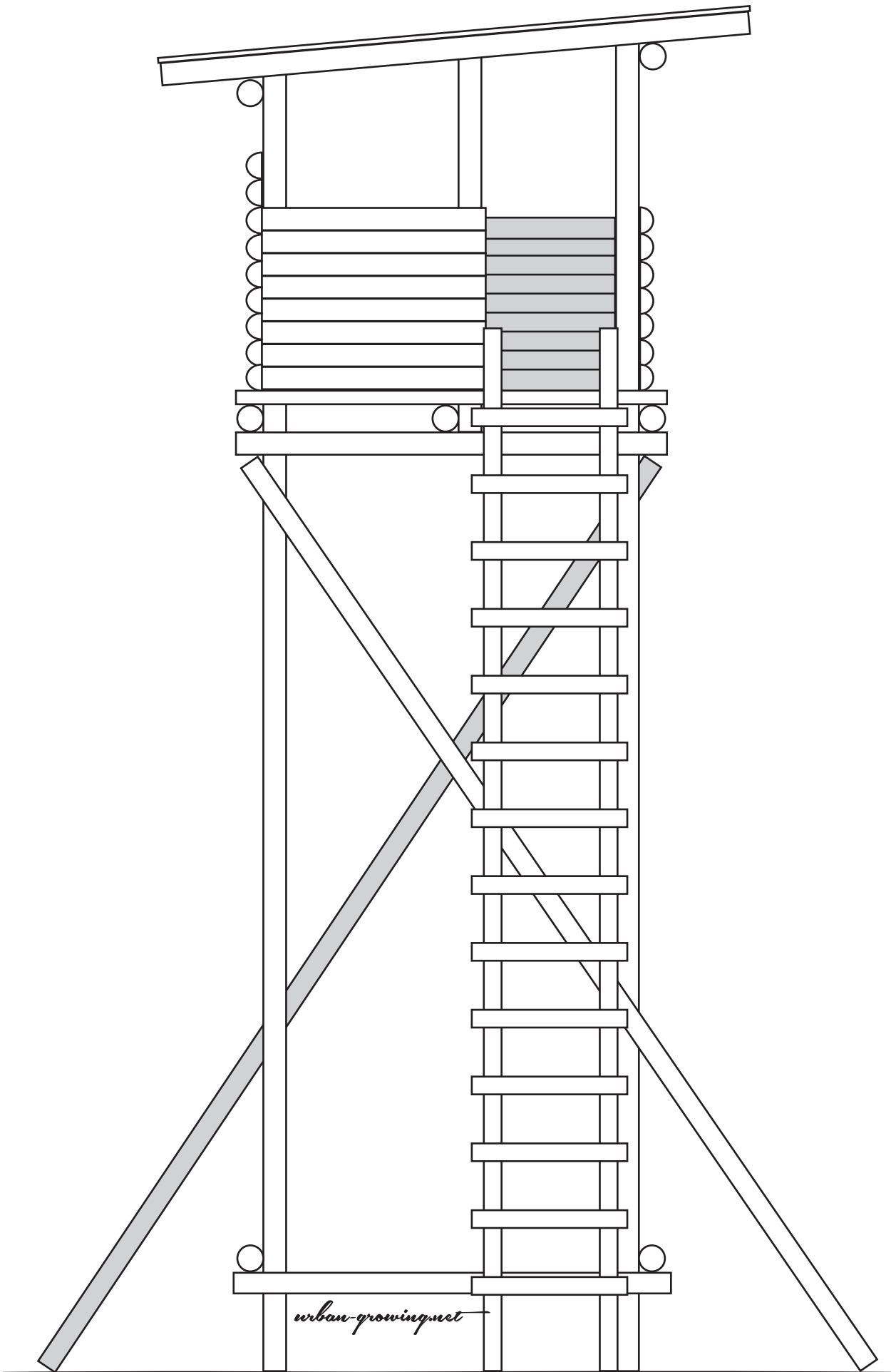
EINFACHER WACHTURM
